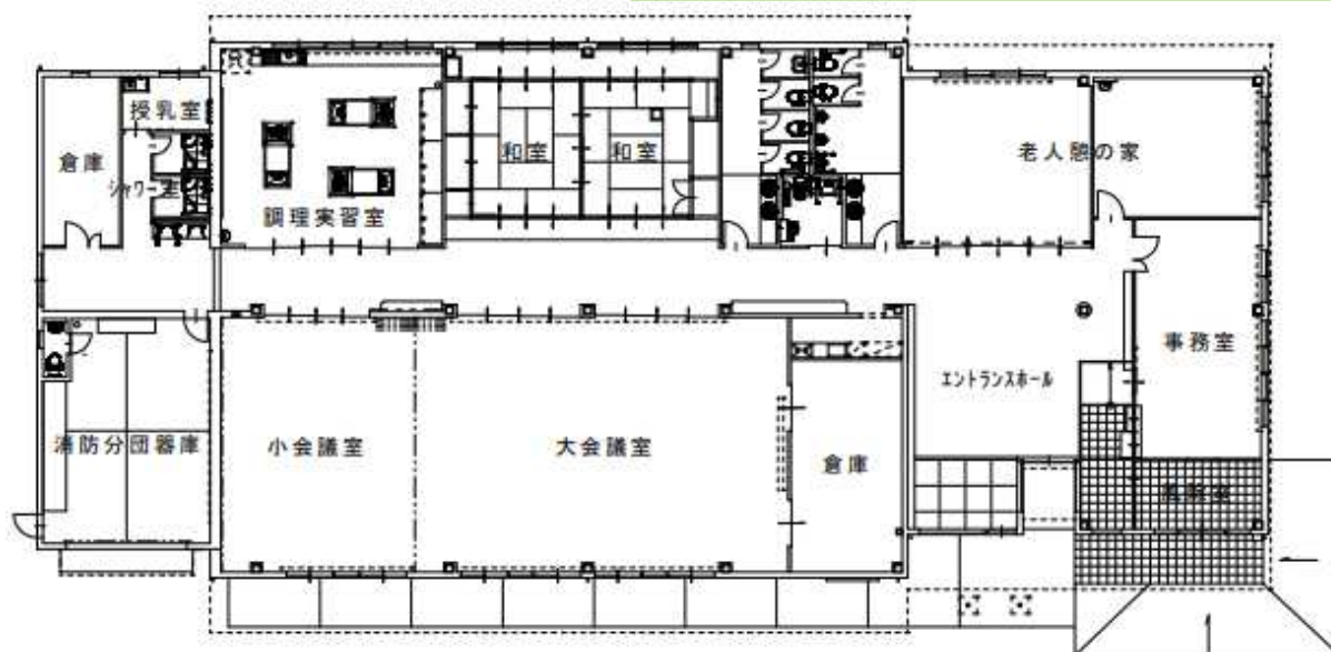
新公民館平面図 平屋建、鉄骨造、一部鉄筋コンクリート造
